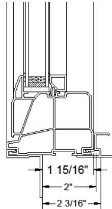
WOOD RETURN & NAIL FIN
