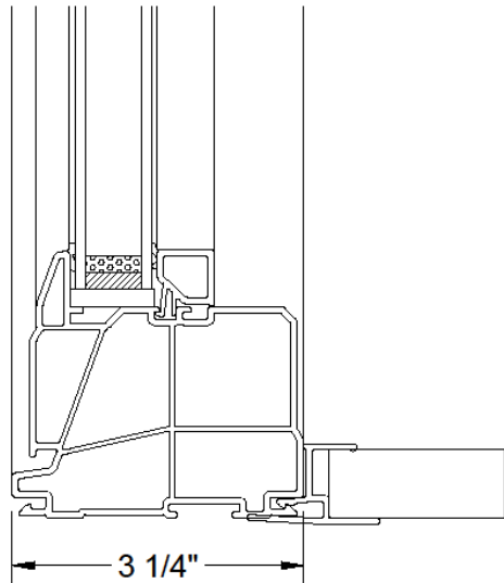
VINYL WRAP JAMB EXTENSION
