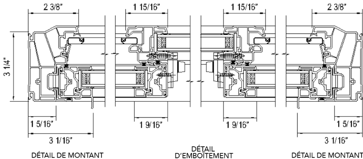
COUPE B-B
