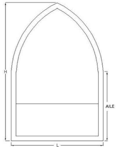
FENÊTRE CATHÉDRALE À UN CHÂSSIS MODÈLE N° 1322
