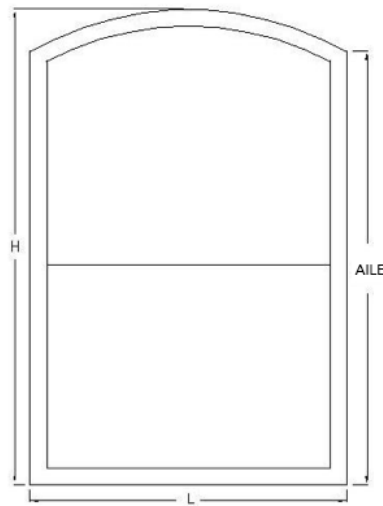
FENÊTRE À HAUT CAMBRÉ À UN CHÂSSIS MODÈLE N° 1321
