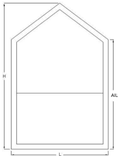
FENÊTRE PENTAGONE À UN CHÂSSIS MODÈLE N° 1324
