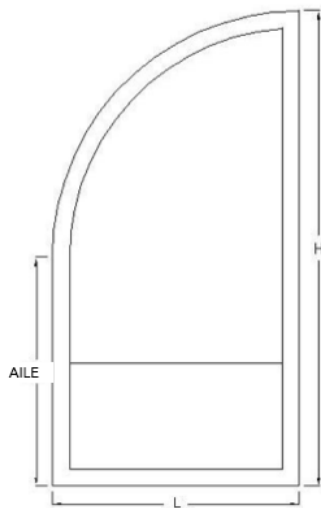
FENÊTRE À QUART D'ARC À UN CHÂSSIS MODÈLE N° 1323
