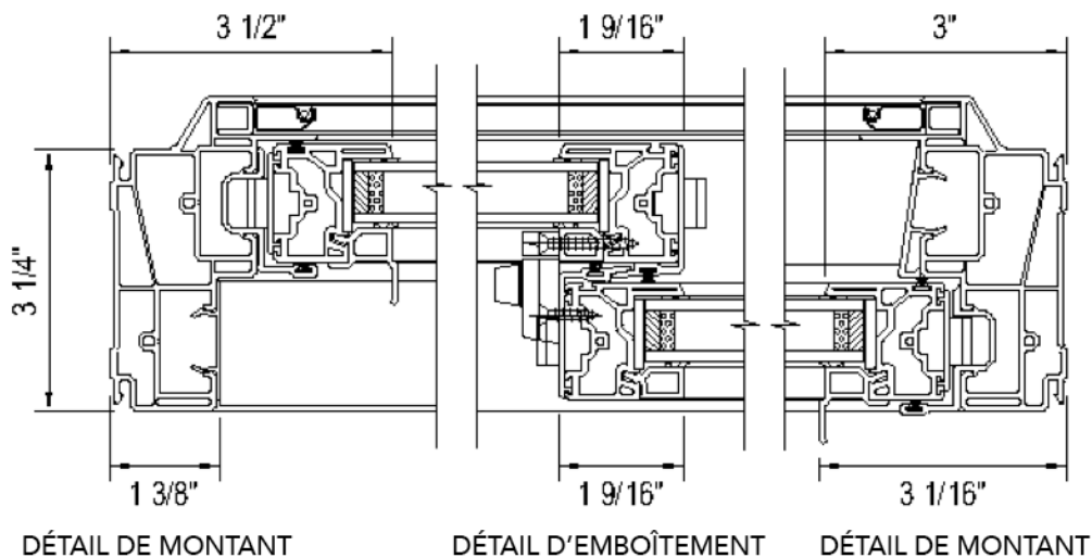
COUPE B-B
