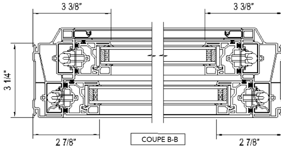
DÉTAIL DE MONTANT
