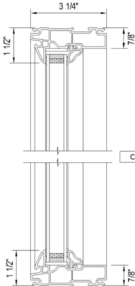
DÉTAIL DE SEUIL
