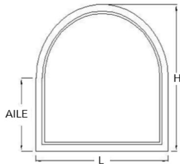
ARC AVEC EXTENSION MODÈLE N° 1028
