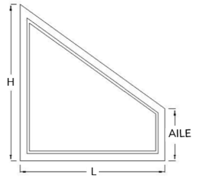
TRAPÈZE MODÈLE N° 1032
