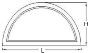
DEMI-ARC MODÈLE N° 1023
