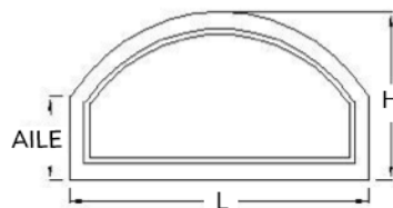
HAUT EN ELLIPSE MODÈLE N° 1026
