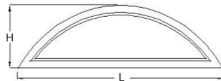
ARCEAU/SOURCIL MODÈLE N° 1025
