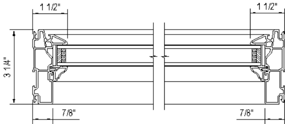
DÉTAIL DE MONTANT
