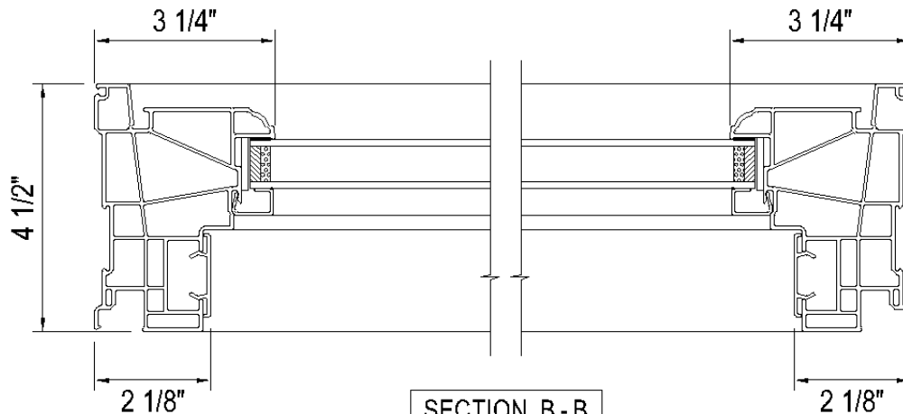
JAMB DETAIL
