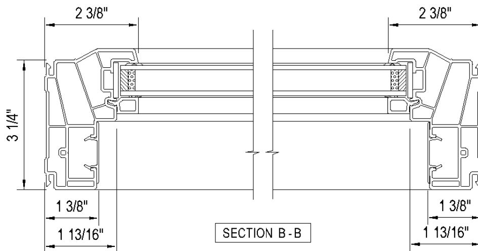
JAMB DETAIL
